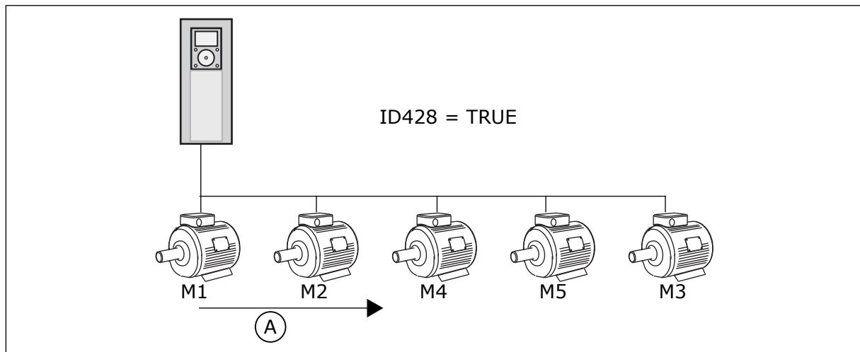
Rys. 83: Logika blokady 3
