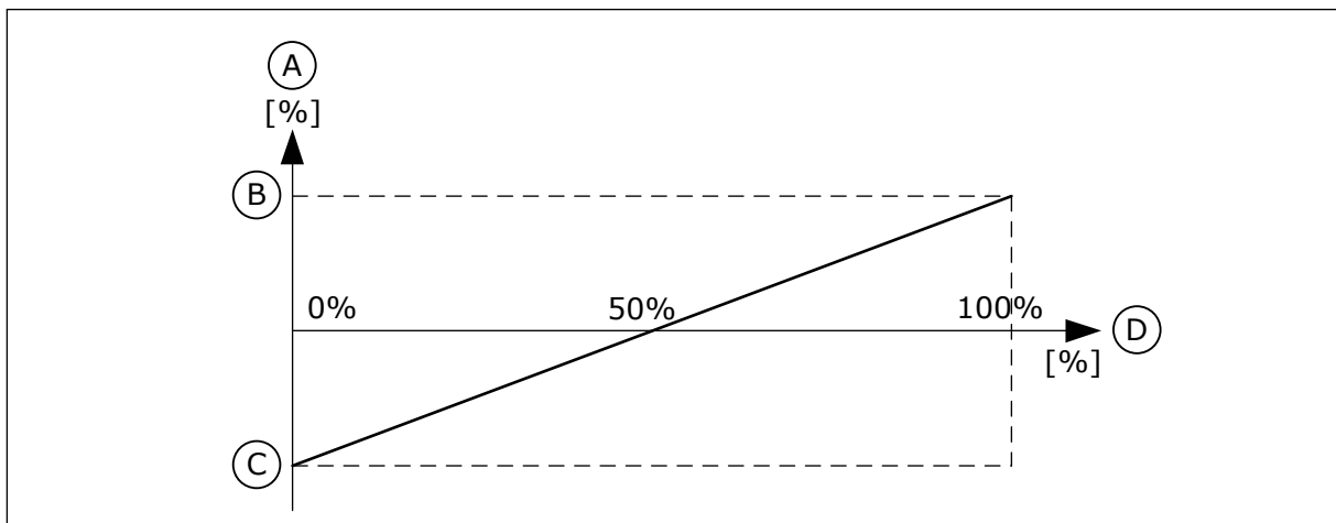
Rys. 34: Skalowanie zadanego sygnału momentu
