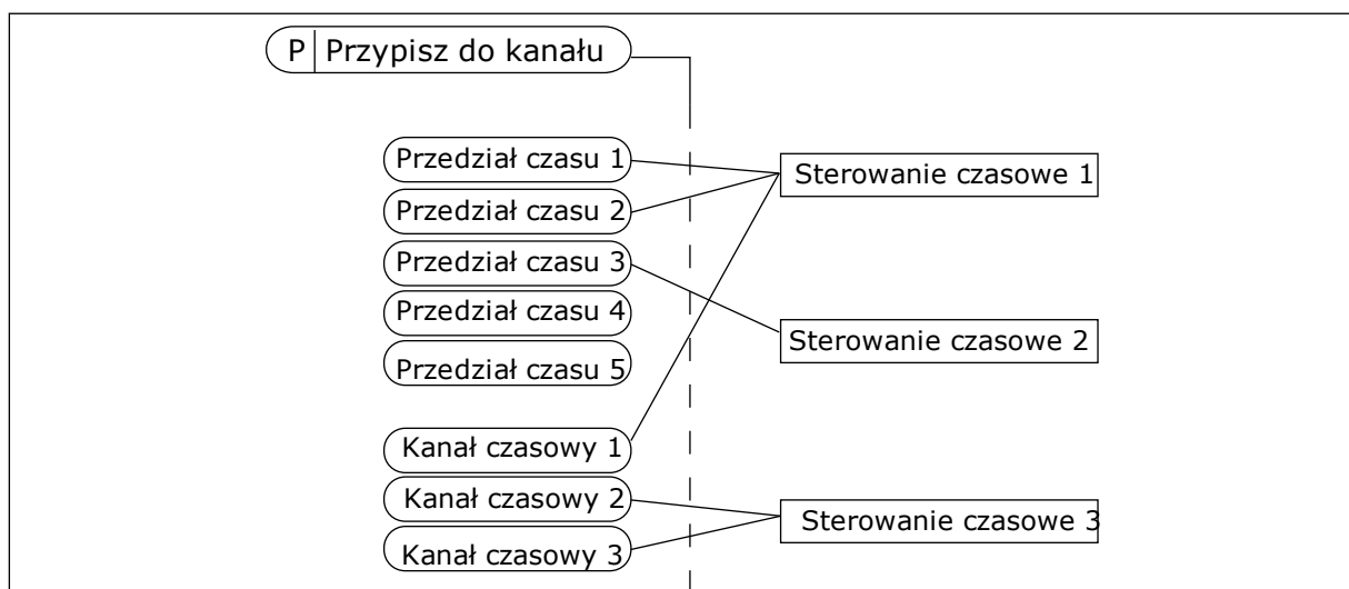
Rys. 64: Sposób przypisywania przedziałów czasu i sterowań czasowych do kanałów czasowych jest bardzo elastyczny. Każdy przedział czasu i każde sterowanie czasowe ma parametr umożliwiający przypisanie do kanału czasowego.
