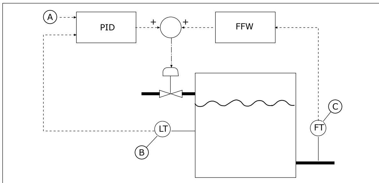
Rys. 71: Sterowanie sprzężeniem wyprzedzającym
