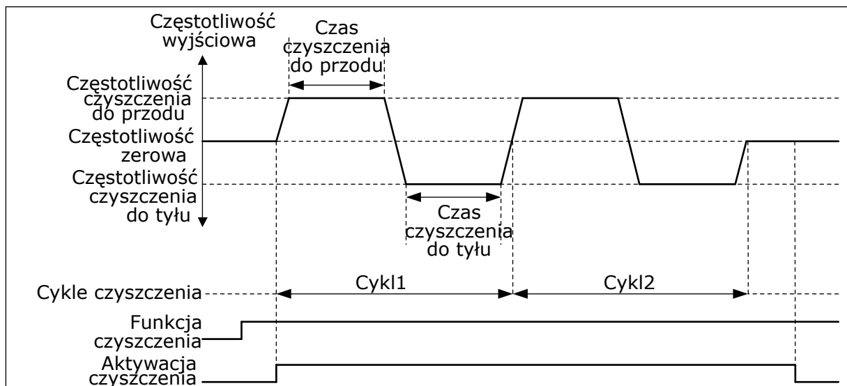
Rys. 91: Funkcja automatycznego czyszczenia
